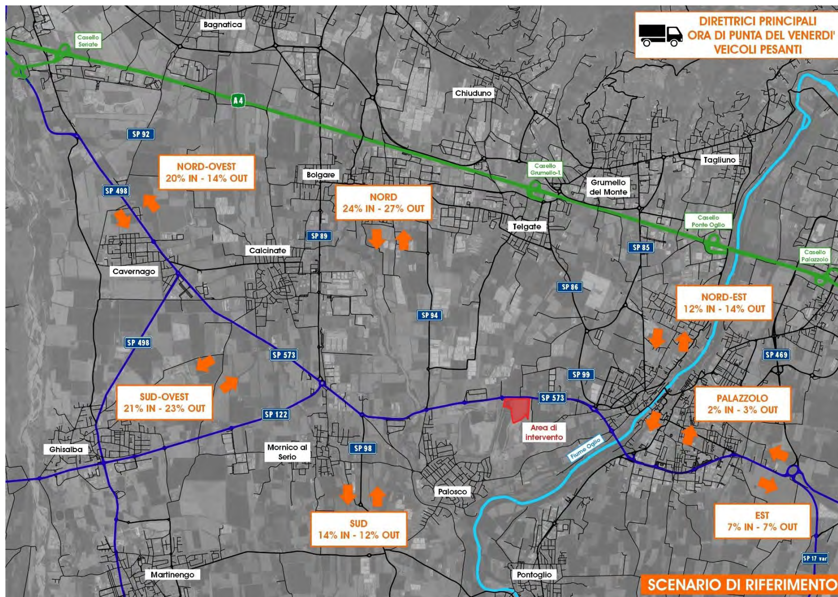
Figura 54 – Scenario di Riferimento – Distribuzione veicoli pesanti nell'ora di punta del venerdì
