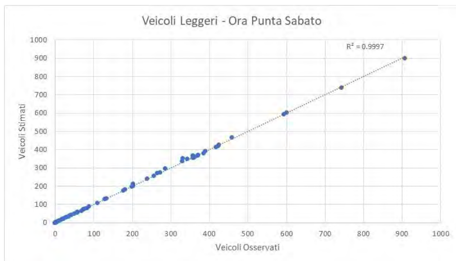
Grafico 9 – Scenario Attuale – Ora di punta del sabato – Confronto flussi osservati e flussi stimati (veicoli leggeri)
