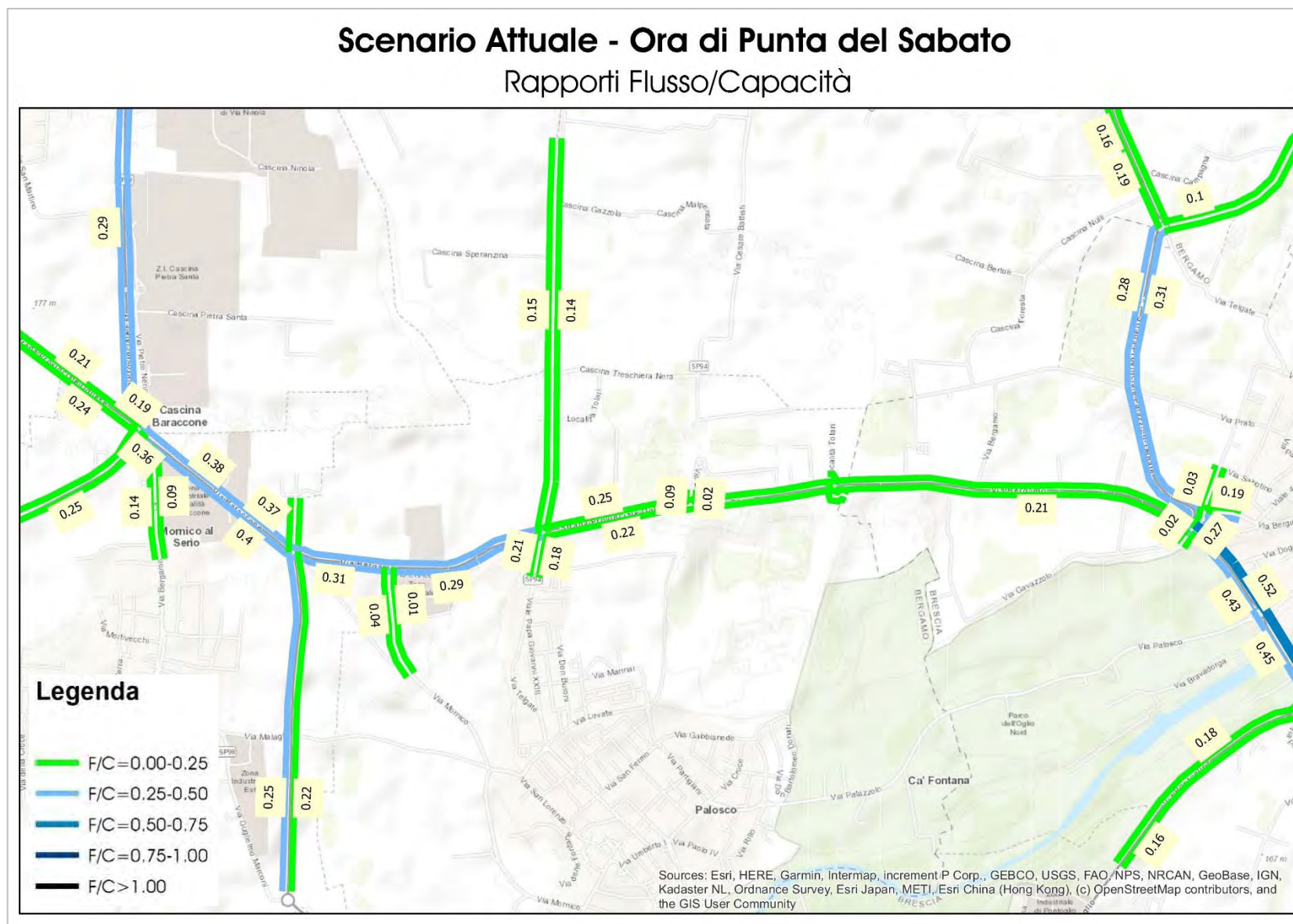
Figura 49 – Scenario Attuale – Ora di punta del sabato – Rapporti Flusso/Capacità
