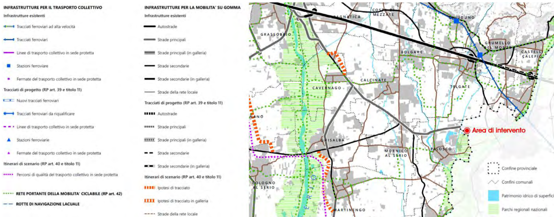
Figura 5 – Estratto del PTCP della provincia di Bergamo – Reti di mobilità
