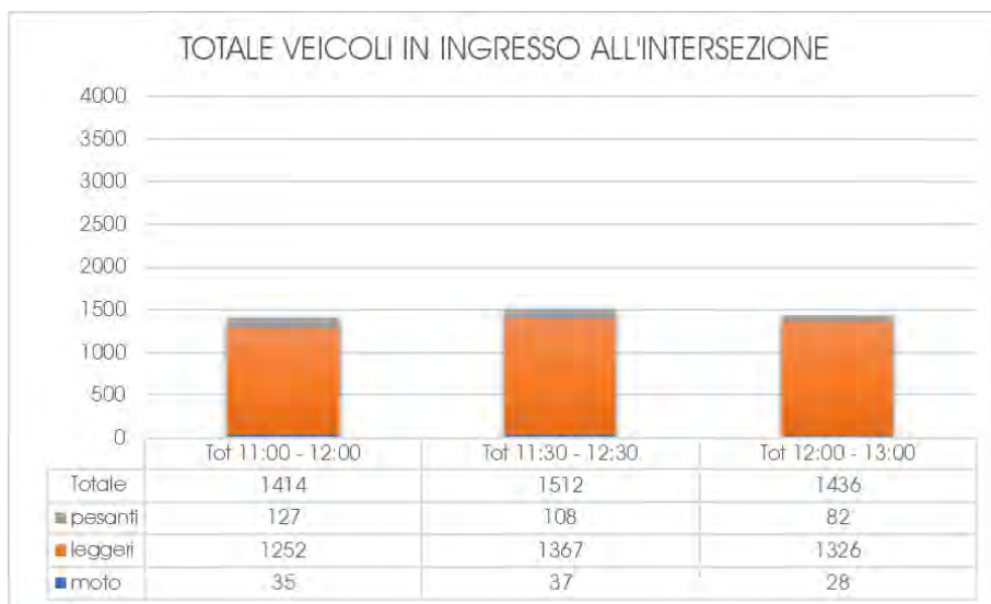
Grafico 39 – Intersezione 2 – Veicoli in ingresso al nodo - Sabato
