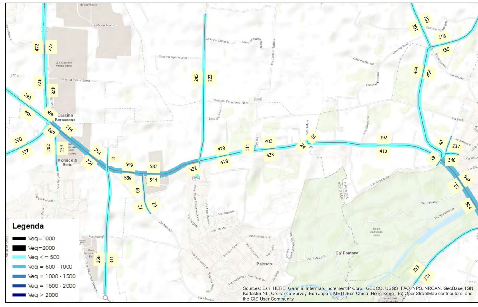
Figura 62 – Scenario di Riferimento – Ora di punta del sabato – Flussogramma area – Veicoli Equivalenti
