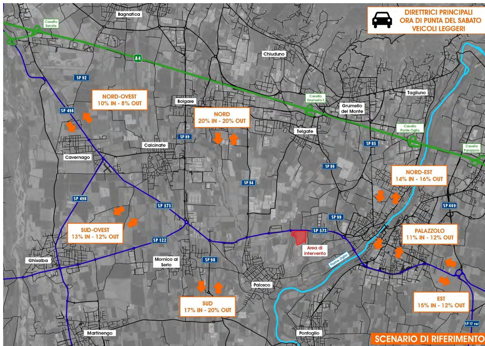
Figura 55 – Scenario di Riferimento – Distribuzione veicoli leggeri nell'ora di punta del sabato
