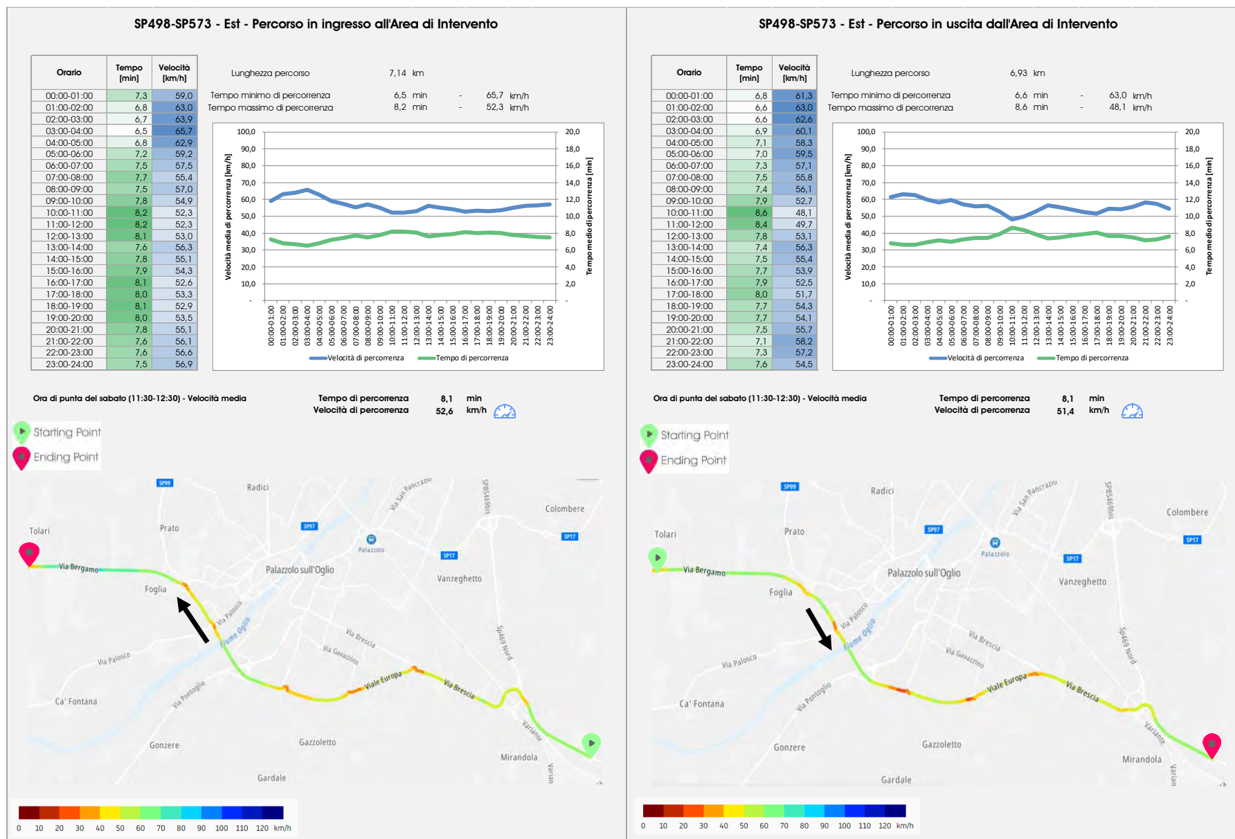
Figura 41 – Analisi dei tempi di percorrenza e delle velocità dai Big Data TomTom – Percorsi ad est dell'area di intervento – Sabato
