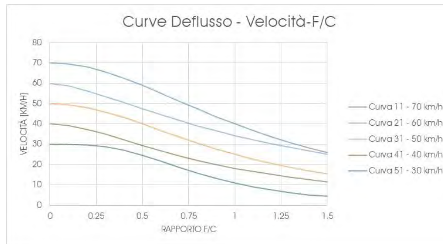
Grafico 5 – Andamento Curve di Deflusso (Velocità – F/C)
