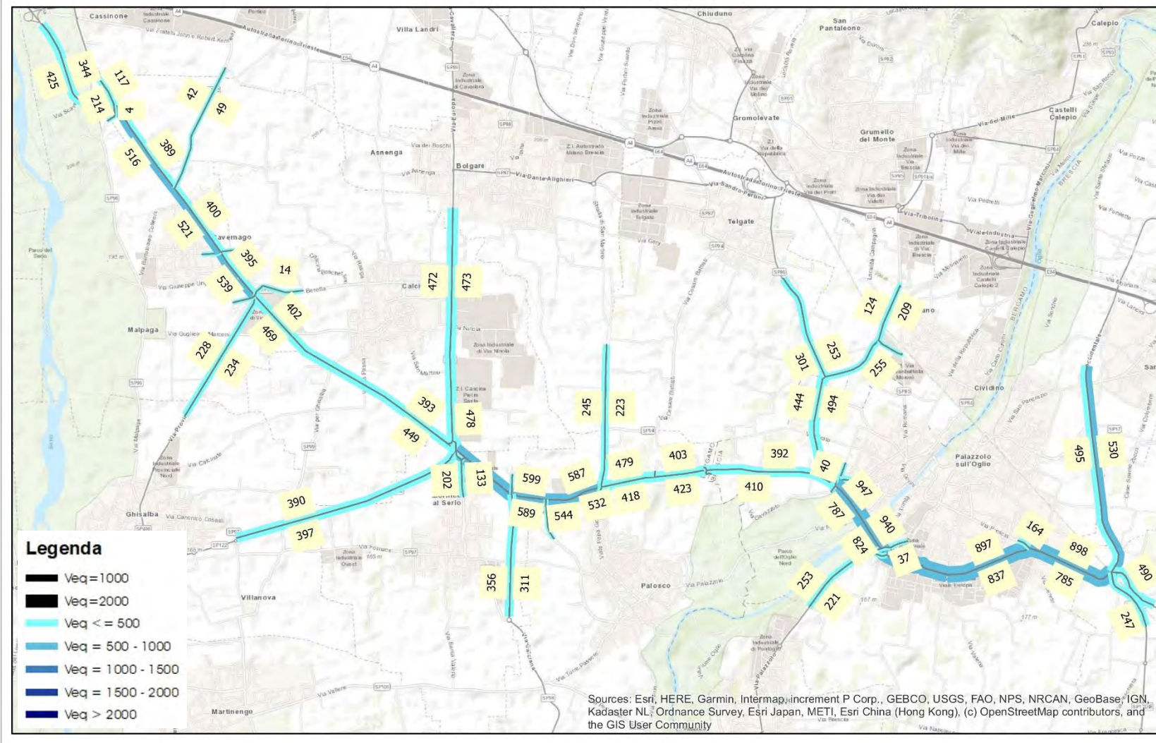
Figura 61 – Scenario di Riferimento – Ora di punta del sabato – Flussogramma area vasta– Veicoli Equivalenti
