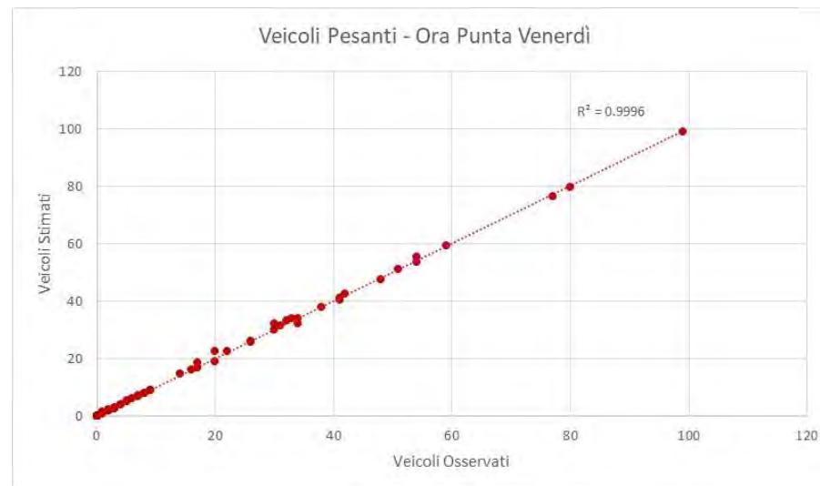
Grafico 8 – Scenario Attuale – Ora di punta del venerdì – Confronto flussi osservati e flussi stimati (veicoli pesanti)
