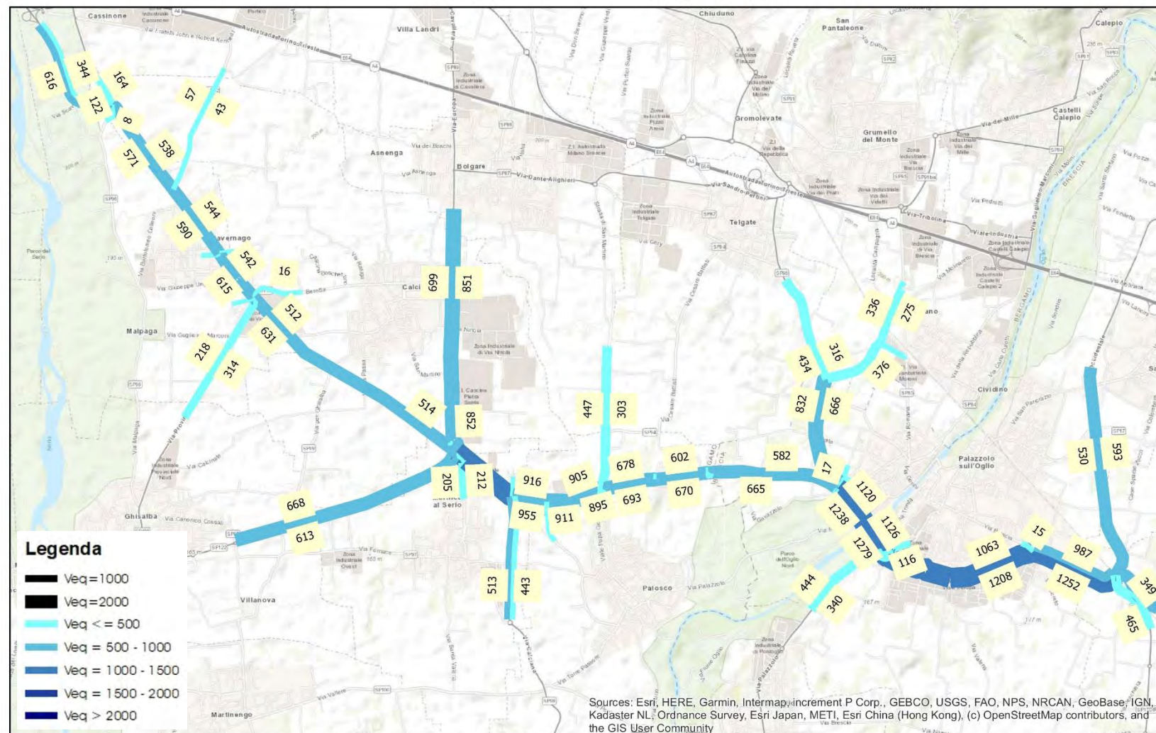
Figura 57 – Scenario di Riferimento – Ora di punta del venerdì – Flussogramma area vasta – Veicoli Equivalenti
