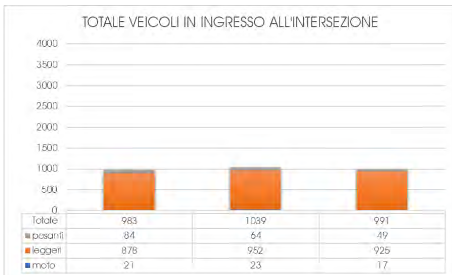
Grafico 15 – Intersezione 1A – Veicoli in ingresso al nodo - Sabato
