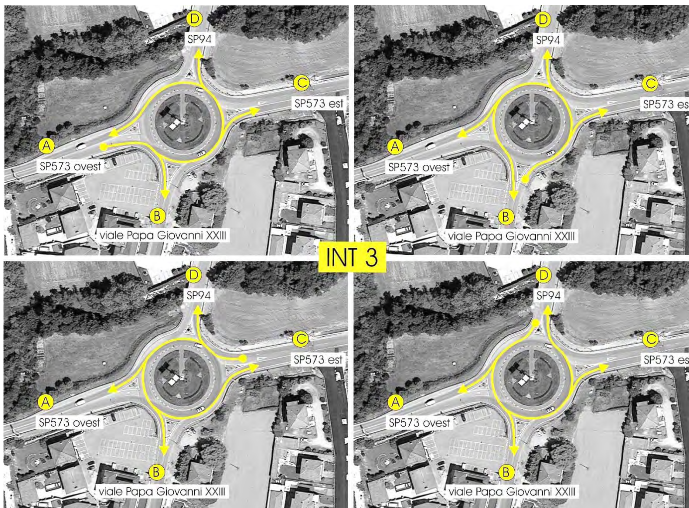
Figura 92 – Intersezione 3 – Manovre rilevate
