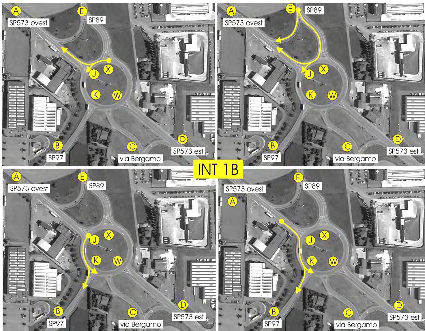
Figura 89 – Intersezione 1B – Manovre rilevate
