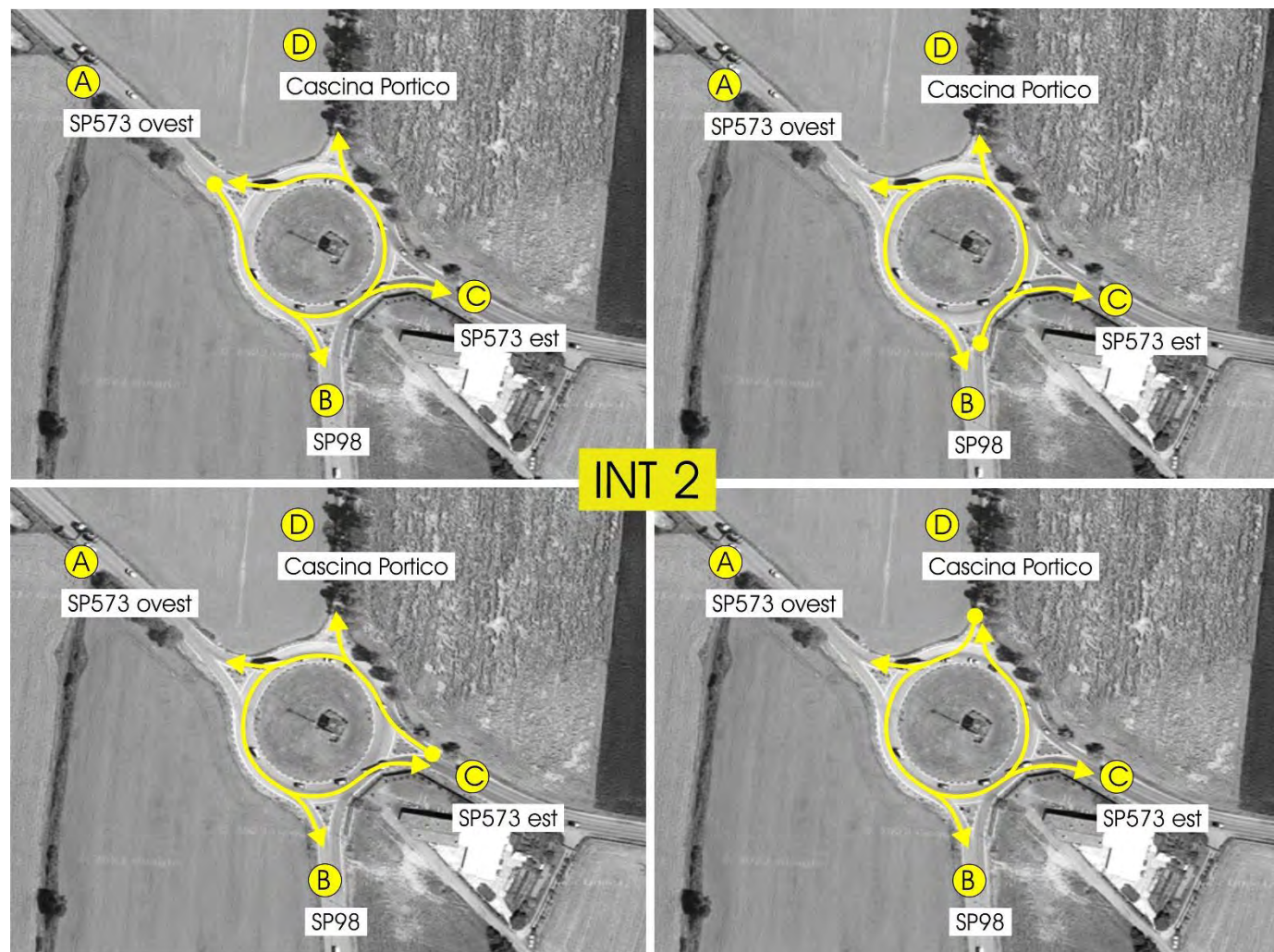
Figura 91 – Intersezione 2 – Manovre rilevate
