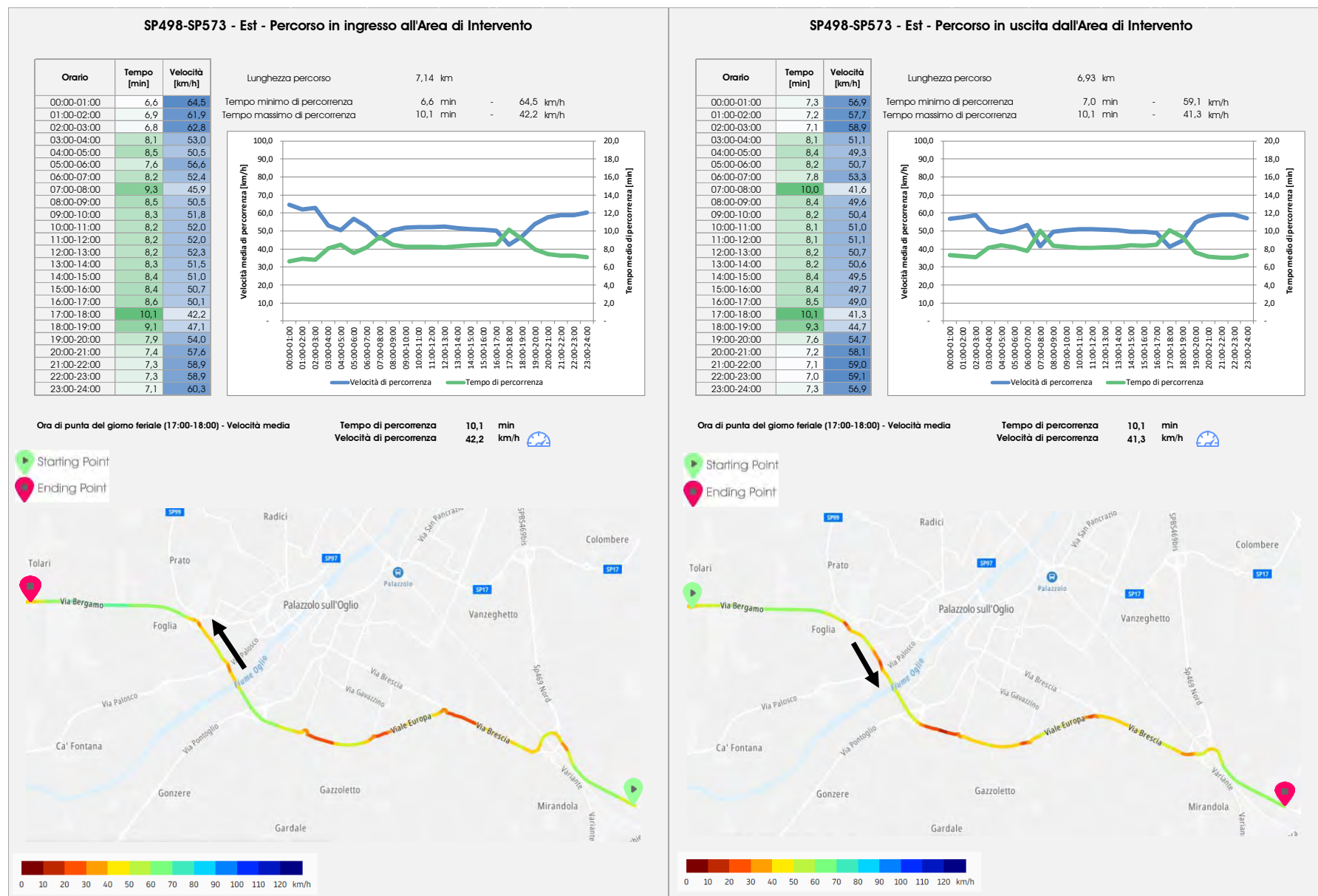
Figura 39 – Analisi dei tempi di percorrenza e delle velocità dai Big Data TomTom – Percorsi ad est dell'area di intervento – Giorno Ferialo
