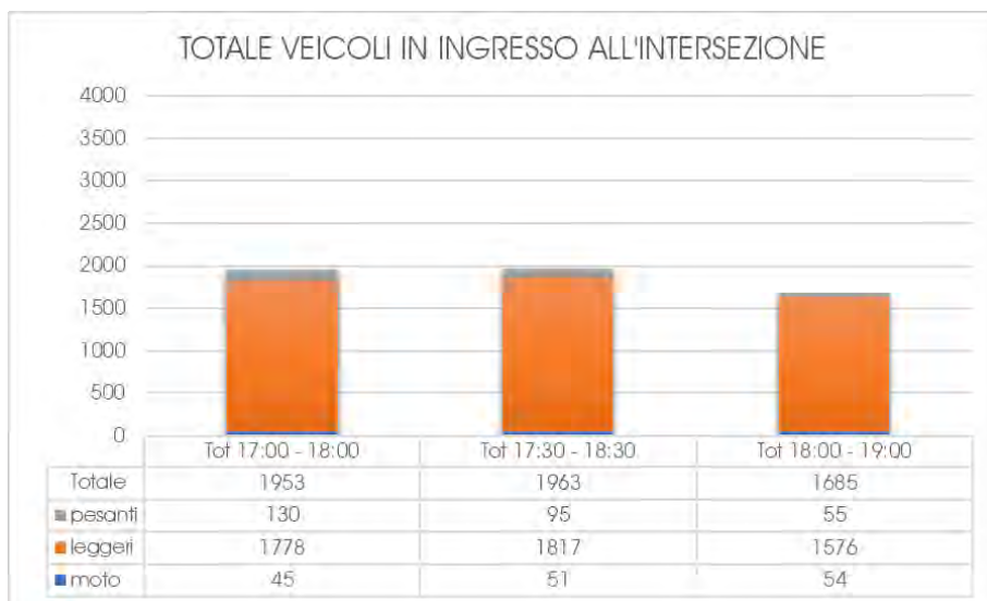
Grafico 43 – Intersezione 3 – Veicoli in ingresso al nodo - Venerdì
