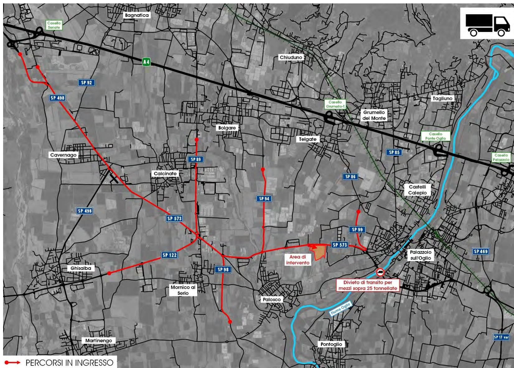
Figura 83 – Percorsi in ingresso all'area di intervento – Veicoli pesanti di cantiere
