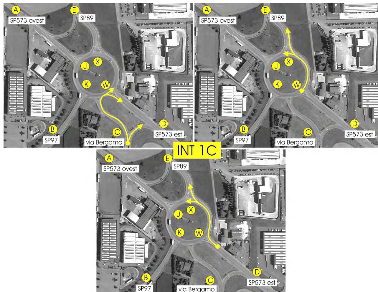
Figura 90 – Intersezione 1C – Manovre rilevate
