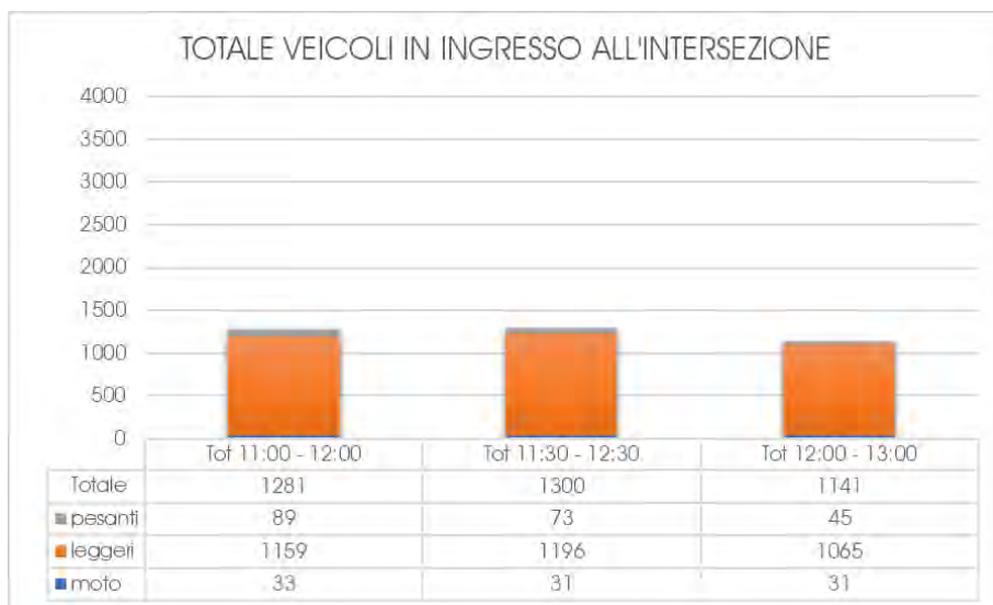
Grafico 47 – Intersezione 3 – Veicoli in ingresso al nodo - Sabato
