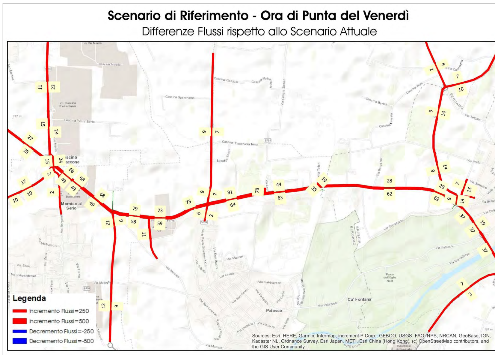
Figura 60 – Scenario di Riferimento – Ora di punta del venerdì – Differenza flussi rispetto allo Scenario Attuale
