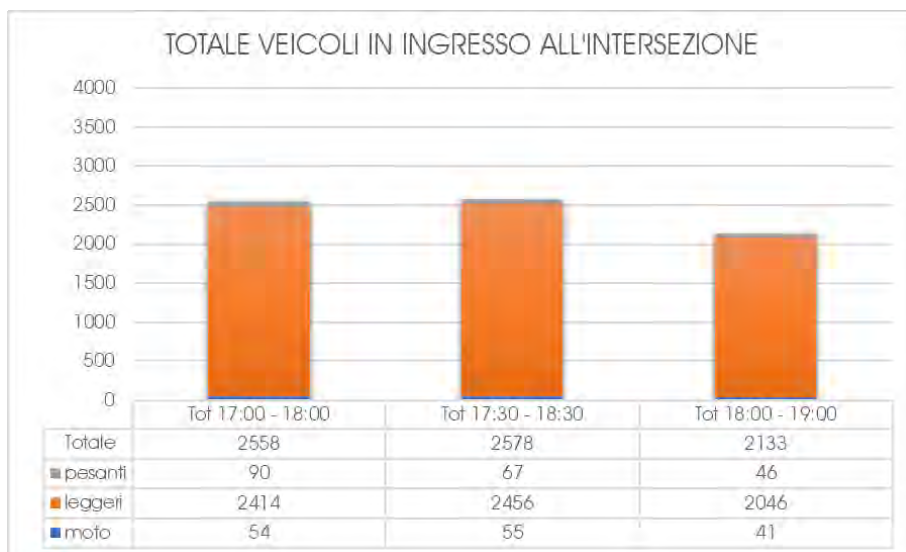
Grafico 67 – Intersezione 5B – Veicoli in ingresso al nodo - Venerdì
