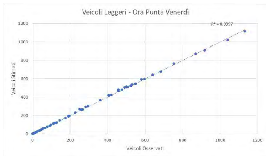
Grafico 7 – Scenario Attuale – Ora di punta del venerdì – Confronto flussi osservati e flussi stimati (veicoli leggeri)
