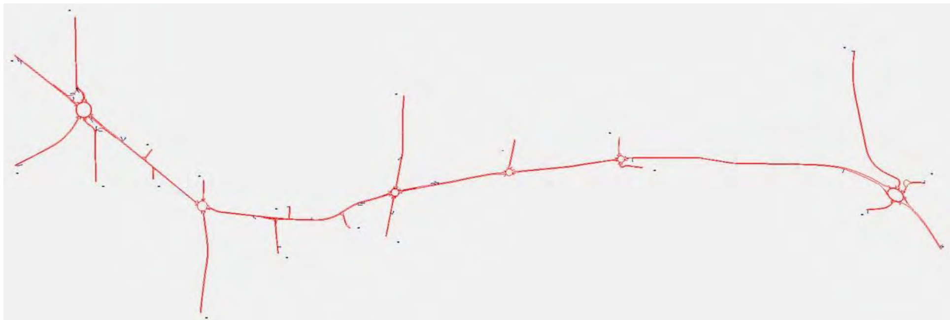
Figura 85 – Rete modello di microsimulazione
