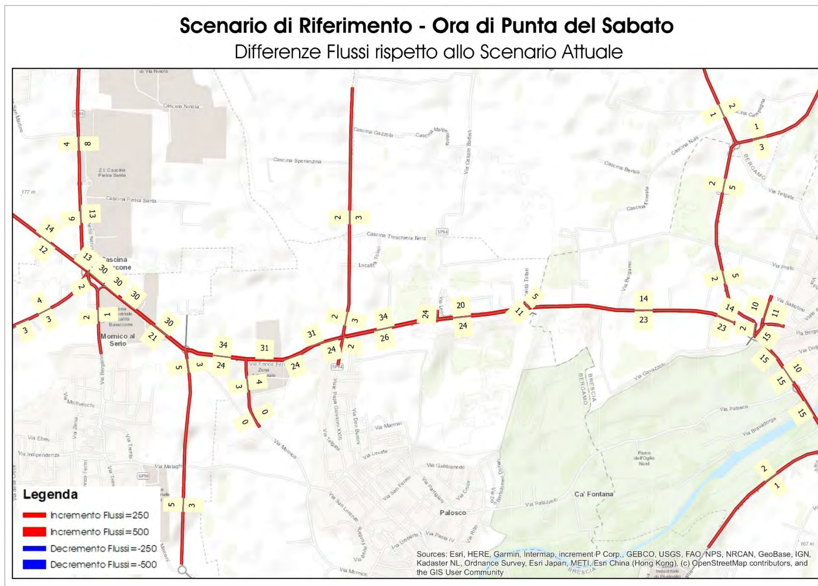
Figura 64 – Scenario di Riferimento – Ora di punta del sabato – Differenza flussi rispetto allo Scenario Attuale
