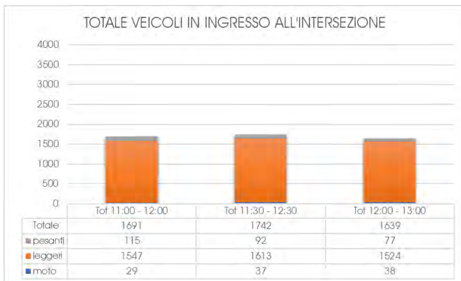
Grafico 23 – Intersezione 1B – Veicoli in ingresso al nodo - Sabato
