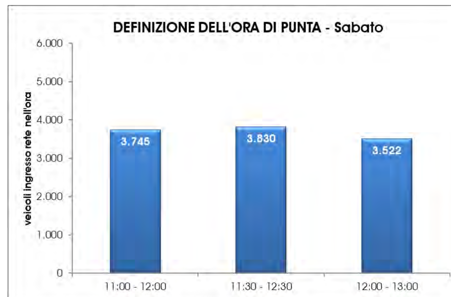
Grafico 4 – Identificazione dell'ora di punta del sabato – Veicoli equivalenti
