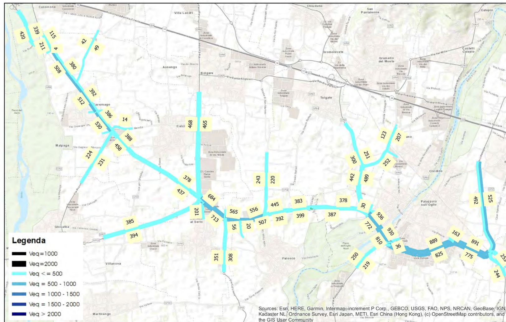
Figura 47 – Scenario Attuale – Ora di punta del sabato – Flussogramma area vasta – Veicoli Equivalenti
