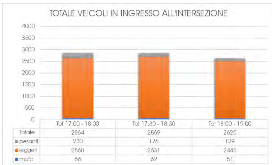
Grafico 19 – Intersezione 1B – Veicoli in ingresso al nodo - Venerdì
