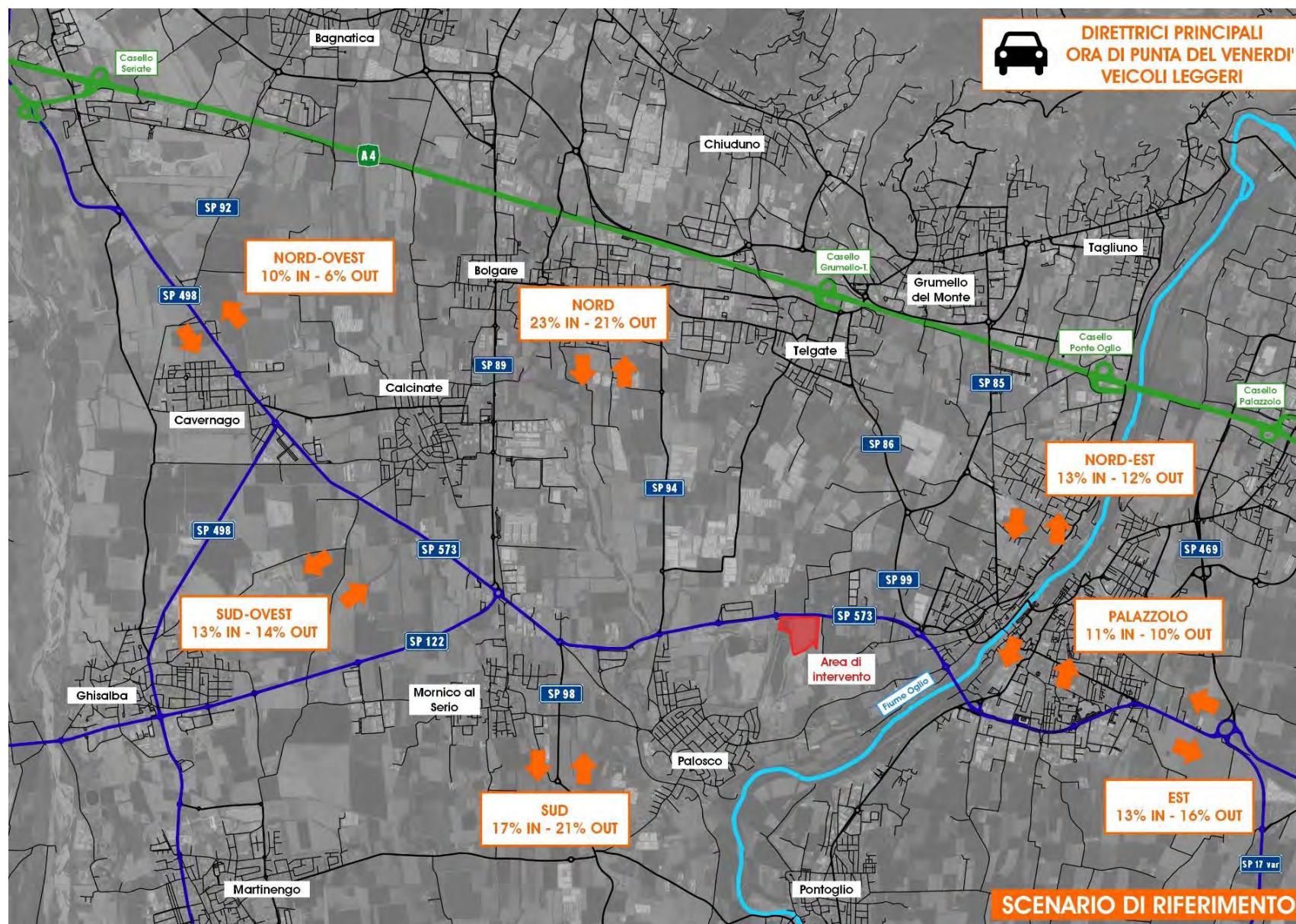
Figura 53 – Scenario di Riferimento – Distribuzione veicoli leggeri nell'ora di punta del venerdì
