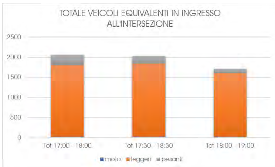
Grafico 44 – Intersezione 3 – Ripartizione modale – Venerdì
