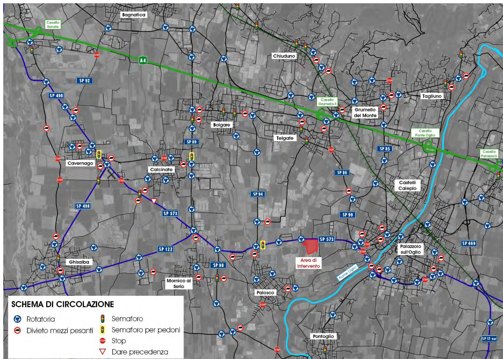
Figura 9 – Schema di circolazione dell'area in esame
