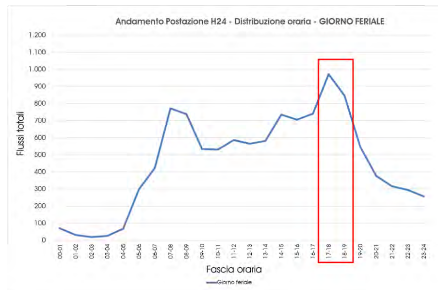
Grafico 1 – Andamento per giorno della settimana e ora del giorno del flusso veicolare bidirezionale (veicoli puri) nel giorno feriale medio
