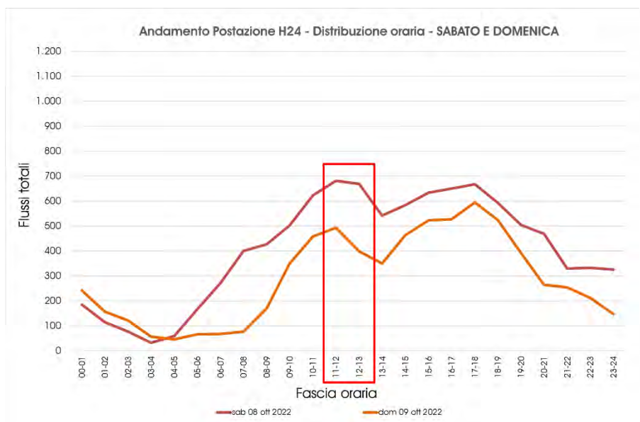
Grafico 2 – Andamento per giorno della settimana e ora del giorno del flusso veicolare bidirezionale (veicoli puri) nel fine settimana
