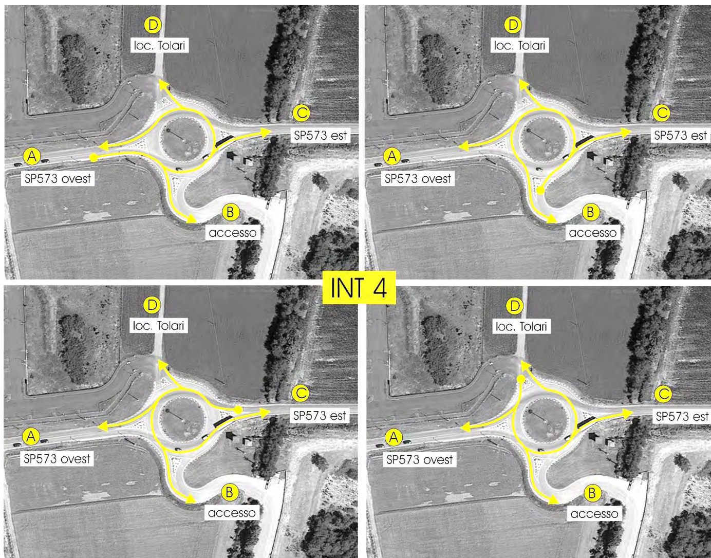
Figura 93 – Intersezione 4 – Manovre rilevate
