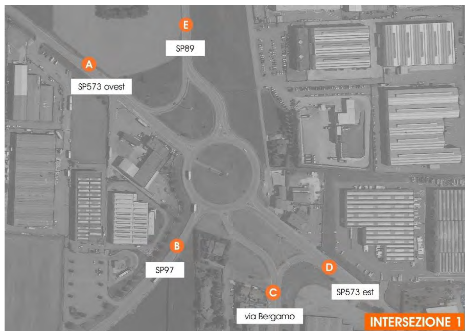
Figura 25 – Intersezione 1: SP573 / SP97 / SP89 / via Bergamo
