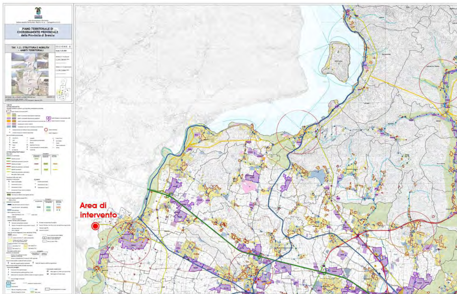
Figura 3 – Estratto del PTCP della provincia di Brescia – Struttura, mobilità e ambiti territoriali
