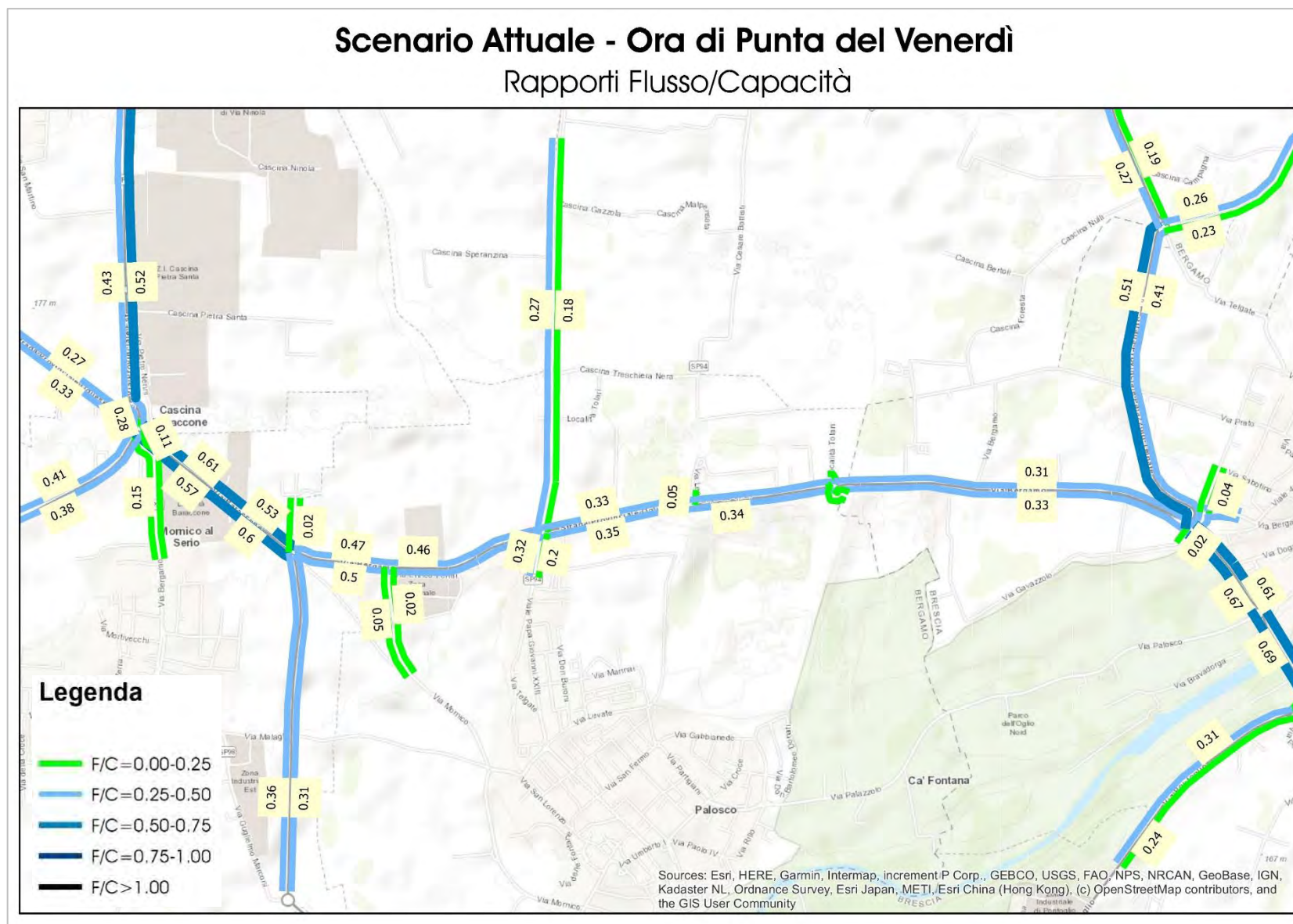
Figura 46 – Scenario Attuale – Ora di punta del venerdì – Rapporti Flusso/Capacità
