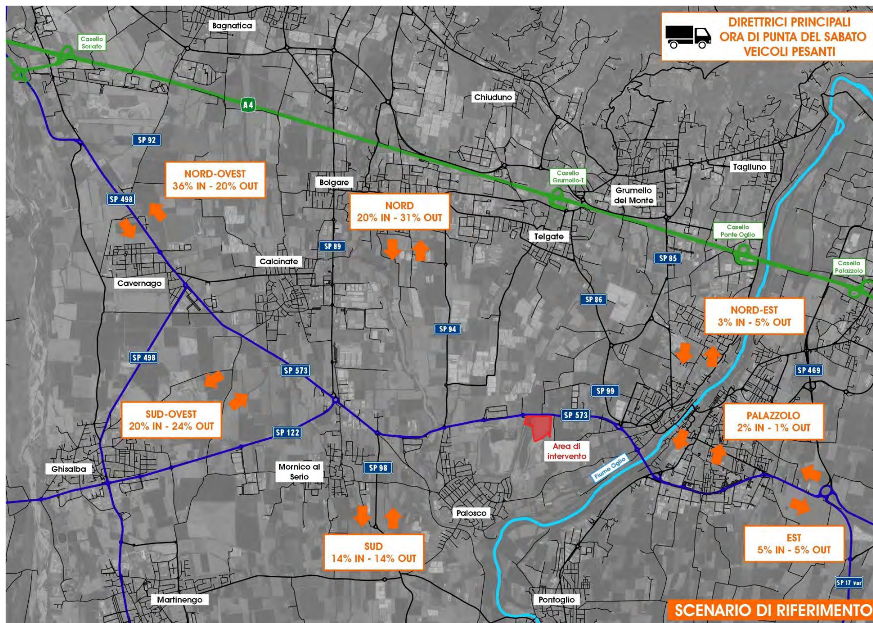
Figura 56 – Scenario di Riferimento – Distribuzione veicoli pesanti nell'ora di punta del sabato
