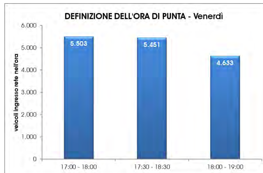
Grafico 3 – Identificazione dell'ora di punta del venerdì – Veicoli equivalenti
