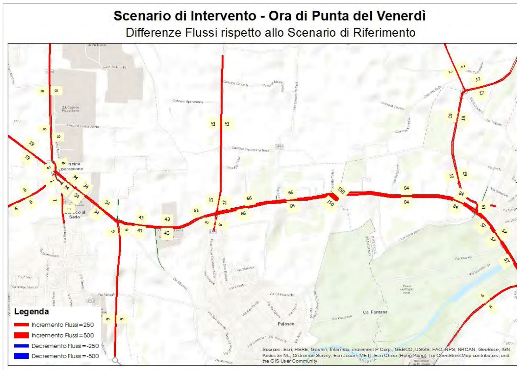
Figura 77 – Scenario di Intervento – Ora di punta del venerdì – Differenza flussi rispetto allo Scenario di Riferimento
