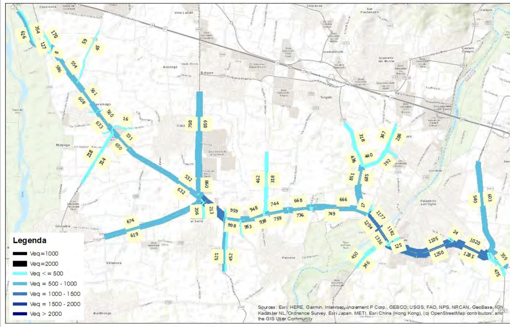
Figura 74 – Scenario di Intervento – Ora di punta del venerdì – Flussogramma area vasta – Veicoli Equivalenti
