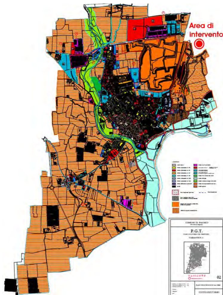
Figura 7 – Estratto del PGT di Palosco – Ambiti di trasformazione territoriale
