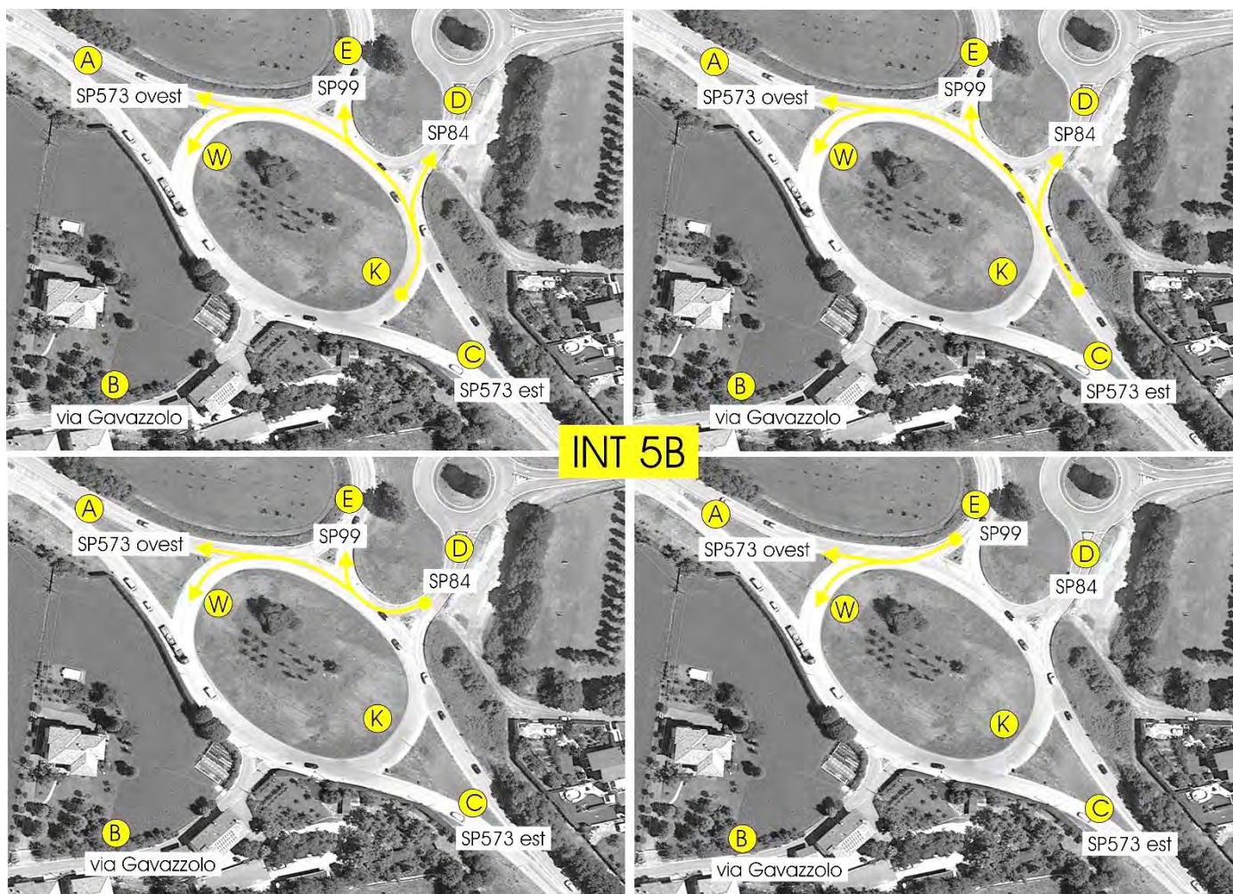
Figura 95 – Intersezione 5B – Manovre rilevate
