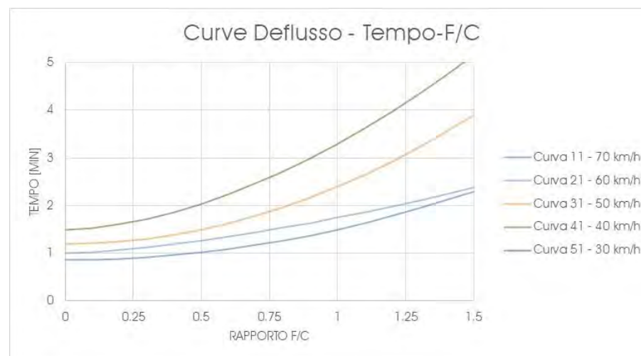
Grafico 6 – Andamento Curve di Deflusso (Tempo – F/C)
