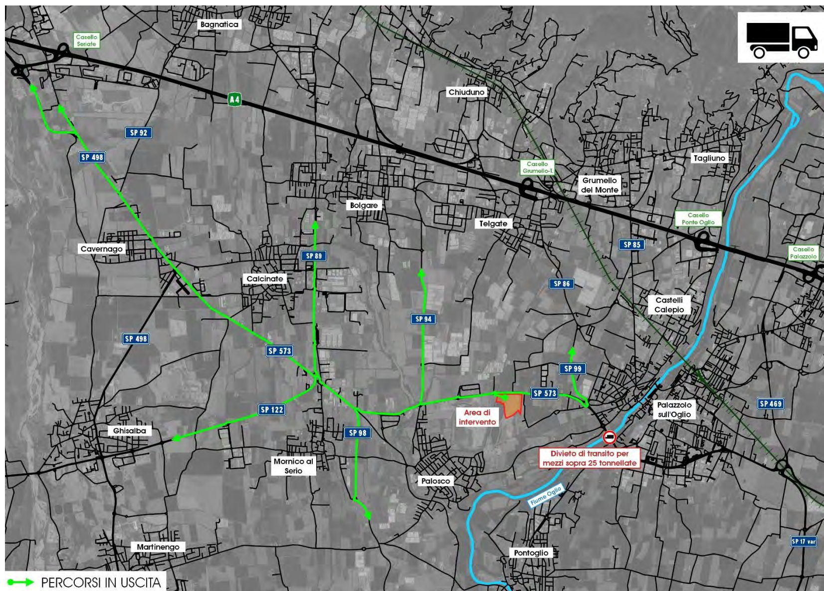
Figura 84 – Percorsi in ingresso all'area di intervento – Veicoli pesanti di cantiere
