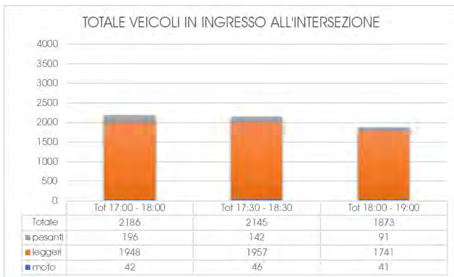
Grafico 35 – Intersezione 2 – Veicoli in ingresso al nodo - Venerdì
