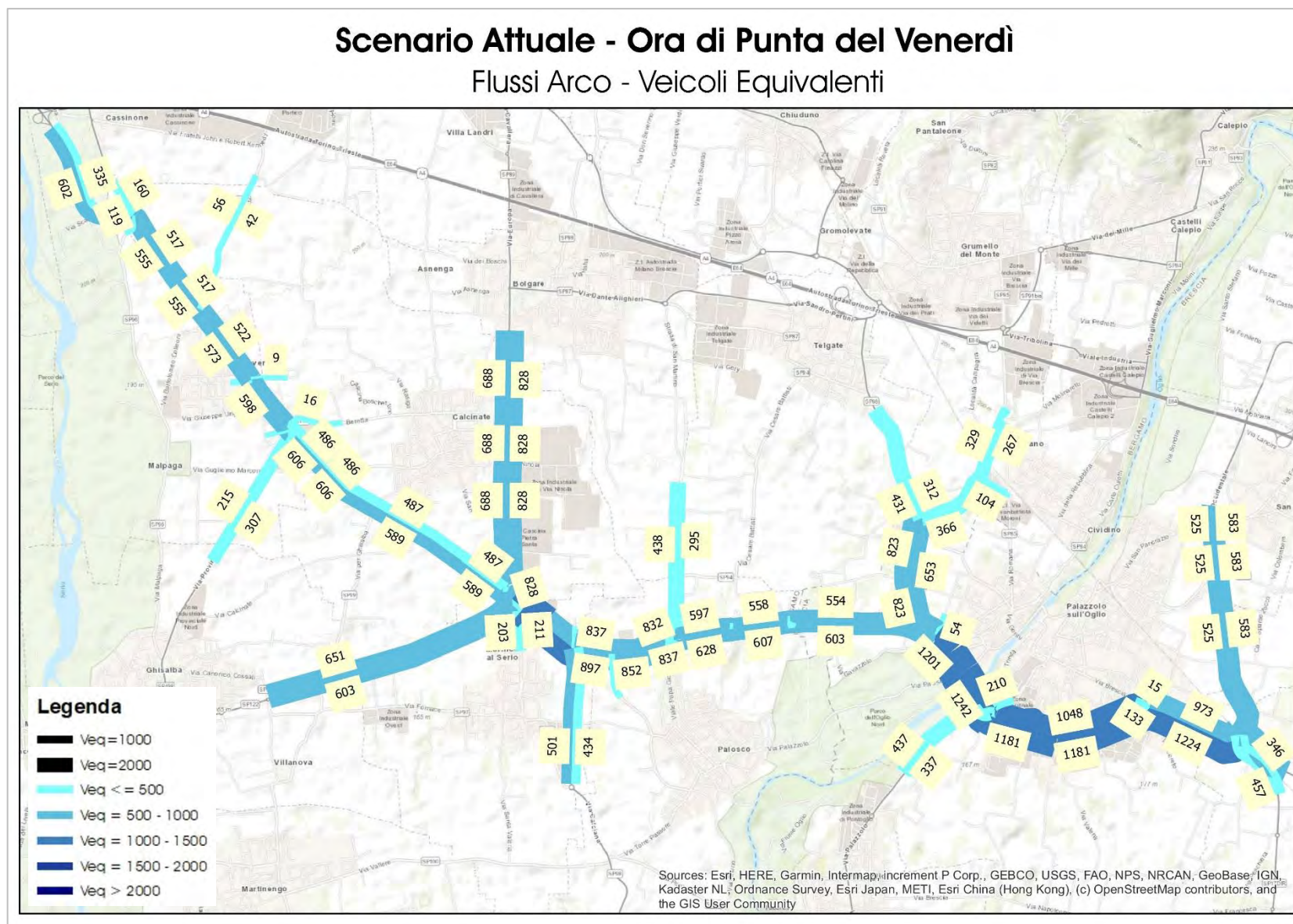
Figura 44 – Scenario Attuale – Ora di punta del venerdì – Flussogramma area vasta – Veicoli Equivalenti
