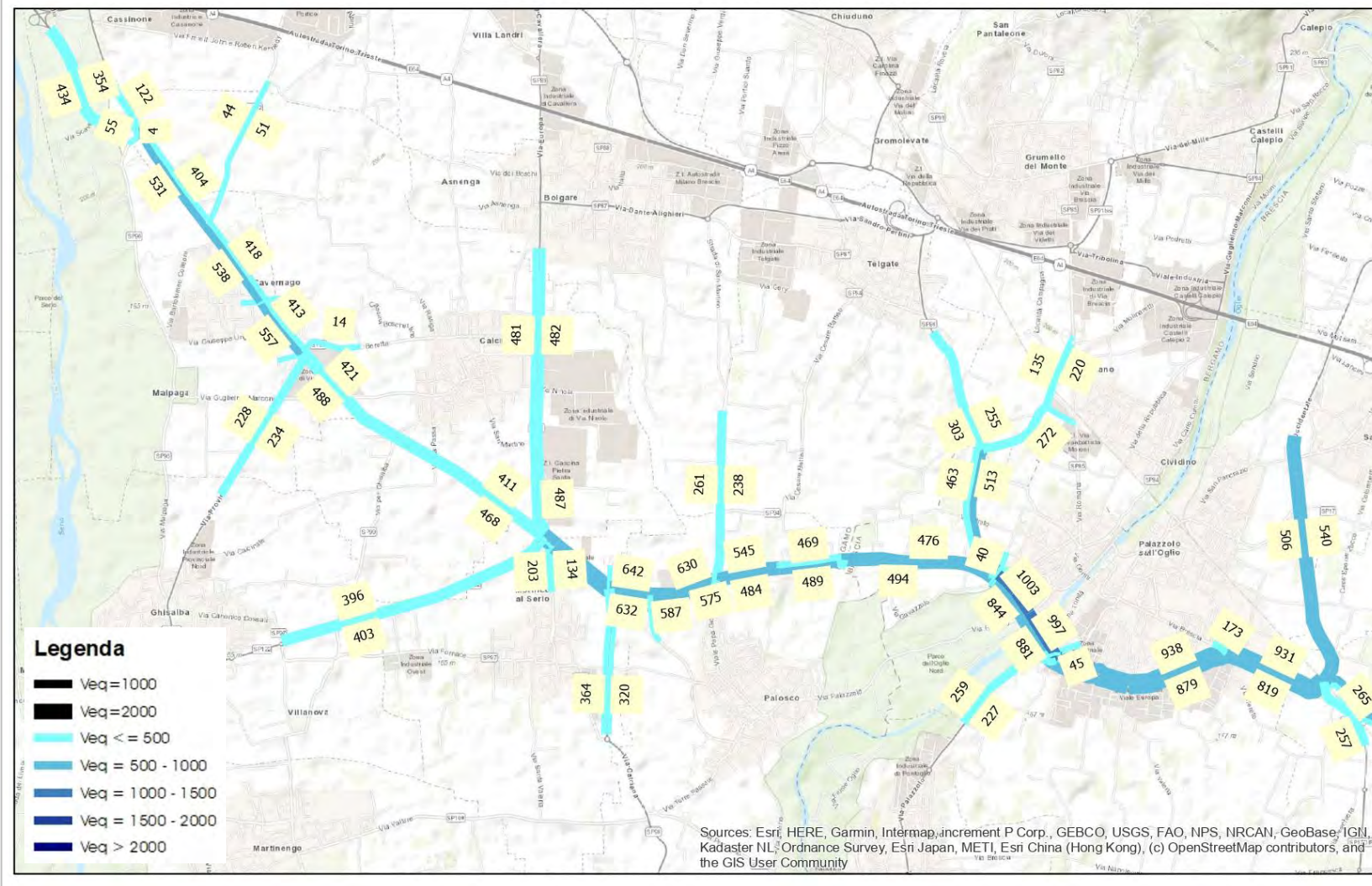
Figura 78 – Scenario di Intervento – Ora di punta del sabato – Flussogramma area vasta– Veicoli Equivalenti
