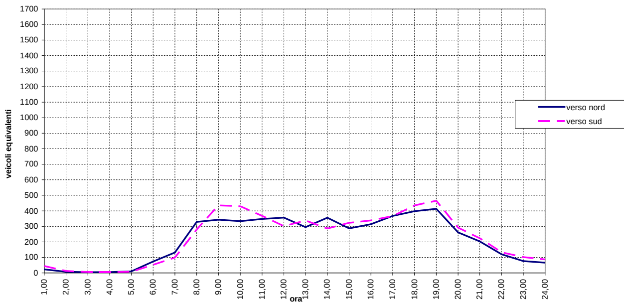
COMUNE DI PALAZZOLO S/O- via Milano Giorno feriale Flusso di traffico omogeneizzato
