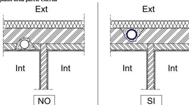
Figura 8: Schemi posizione impianti nella parete esterna
