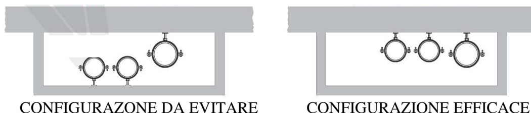
Figura 6: Posizione impianti all'interno del cavedio
