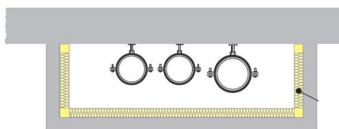
Figura 5: Cavedio insonorizzato per l'inserimento delle tubazioni
