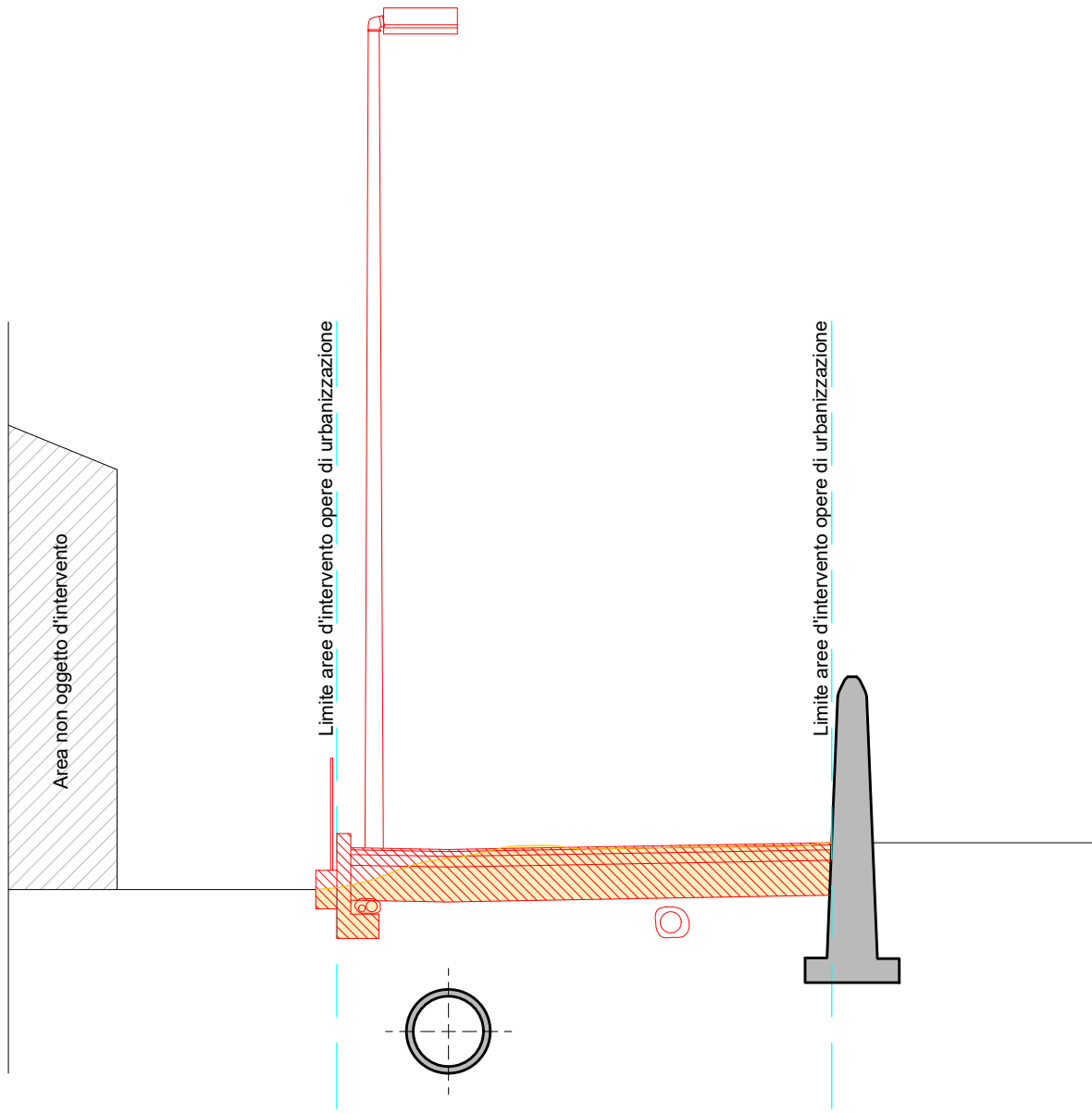
SEZIONE C-C - Sovrapposizione - Scala 1:100
