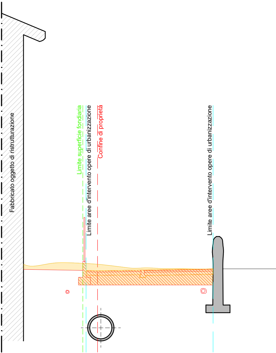
SEZIONE F-F - Sovrapposizione - Scala 1:100
