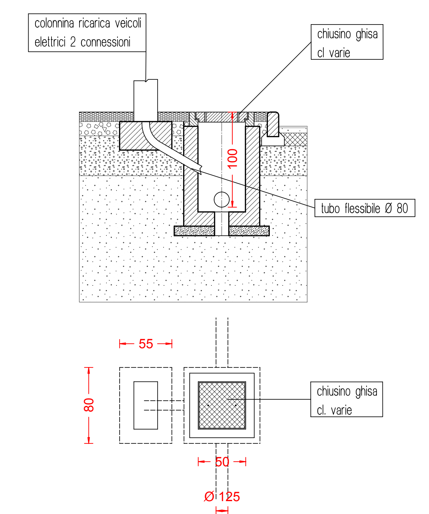
PARTICOLARE COLONNINA RICARICA AUTOVEICOLI ELETTTRICI scala 1:25
