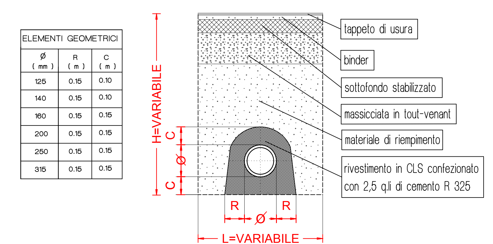
PARTICOLARE POSA CAVIDOTTI scala 1:25
