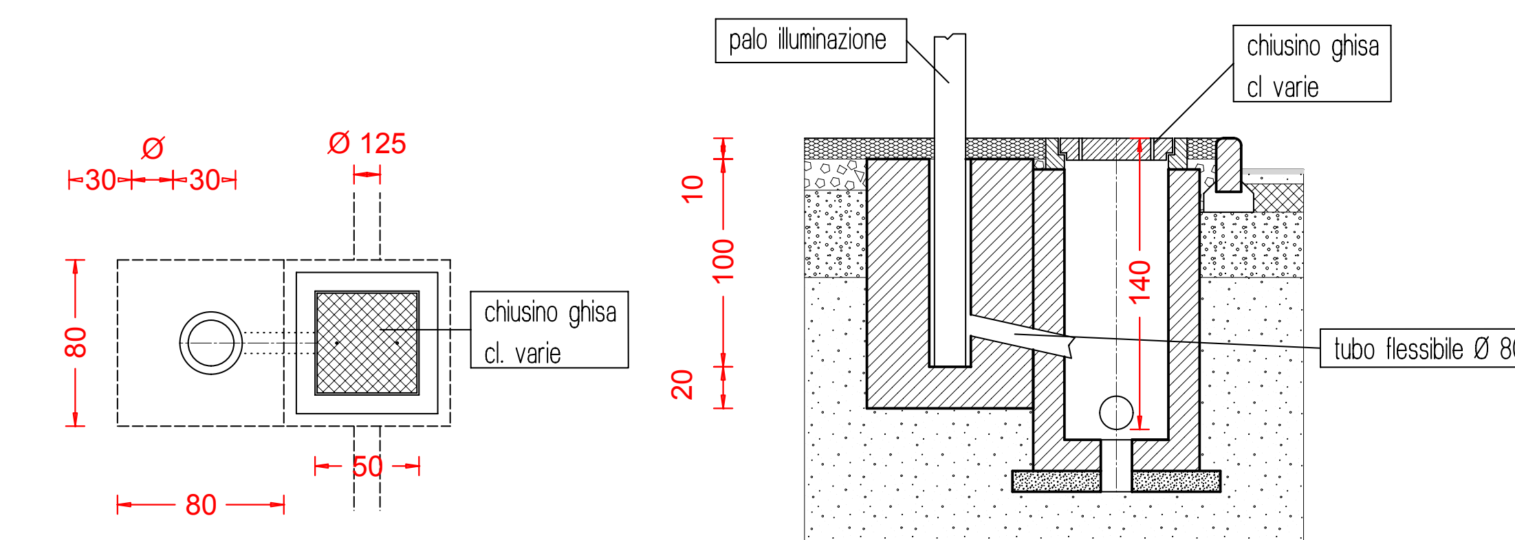
PARTICOLARE PLINTO E POZZETTO ISPEZIONE ILLUMINAZIONE PUBBLICA scala 1:25
