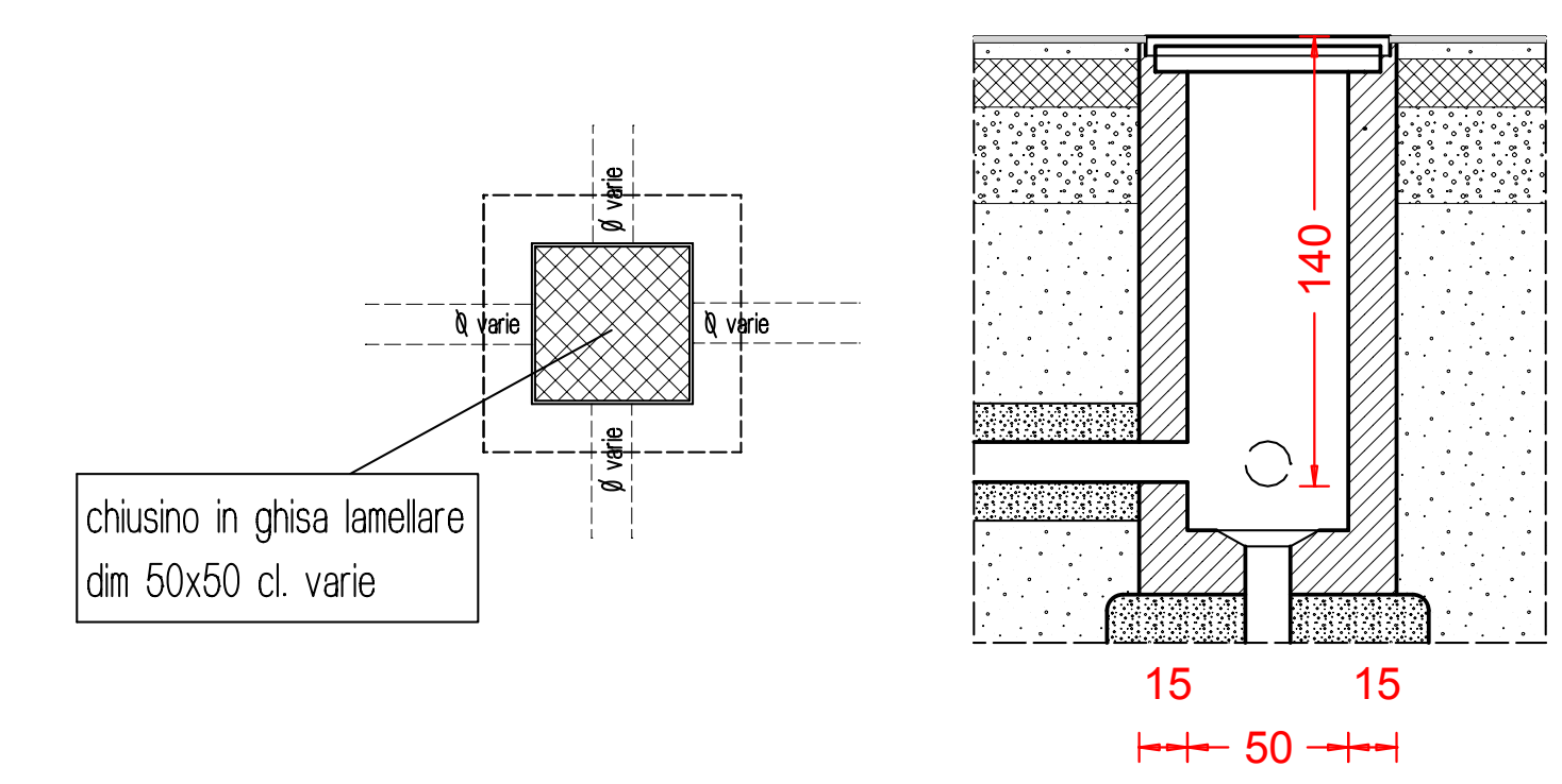
PARTICOLARE POZZETTO ISPEZIONE scala 1:25
