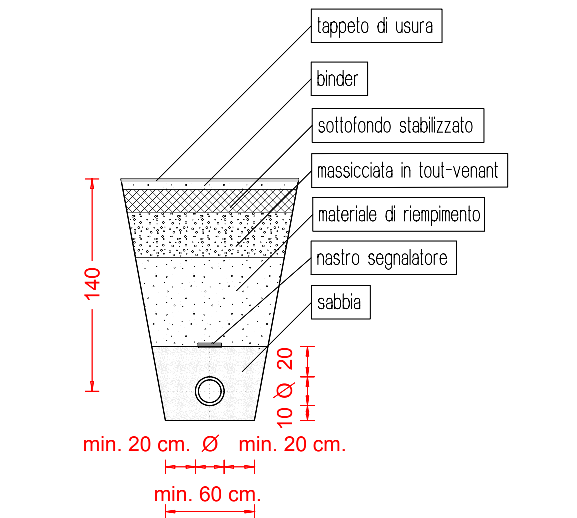
PARTICOLARE POSA CONDOTTA ACQUEDOTTO scala 1:25
