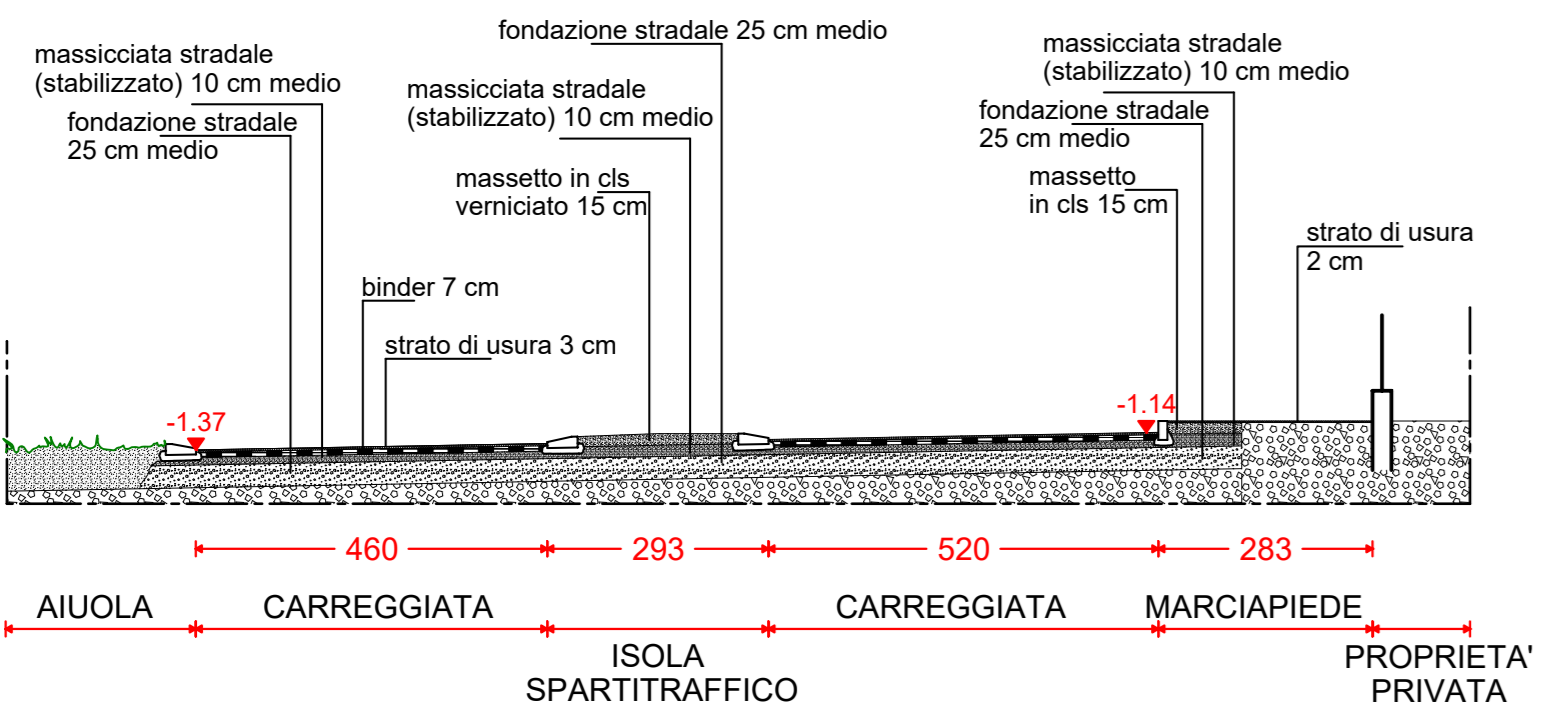
SEZIONE AA DI PROGETTO INCROCIO VIA BERGAMO VIA IV NOVEMBRE scala 1:100
