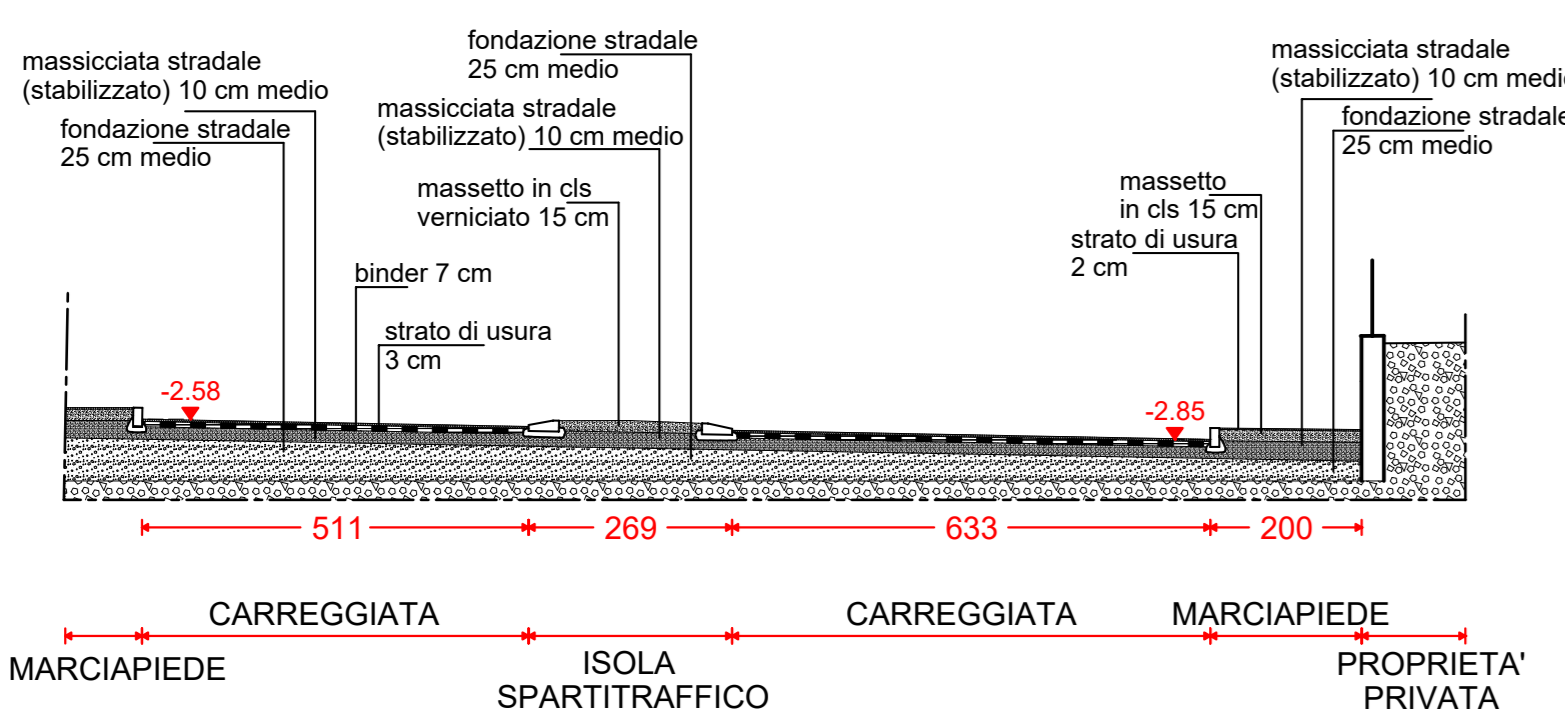
SEZIONE CC DI PROGETTO INCROCIO VIA BERGAMO VIA IV NOVEMBRE scala 1:100
