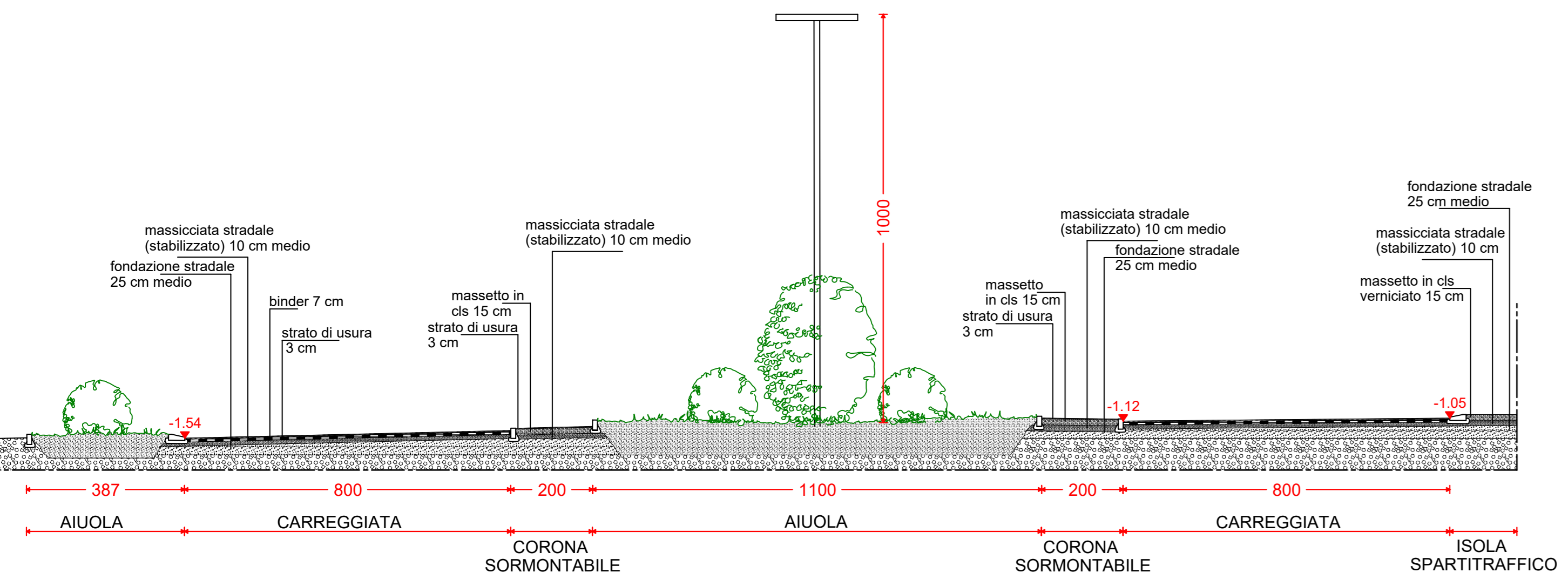
SEZIONE BB DI PROGETTO INCROCIO VIA BERGAMO VIA IV NOVEMBRE scala 1:100
