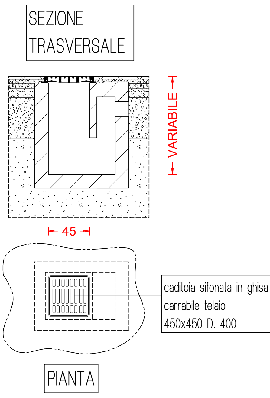
PARTICOLARE CADITOIA STRADALE scala 1:25
