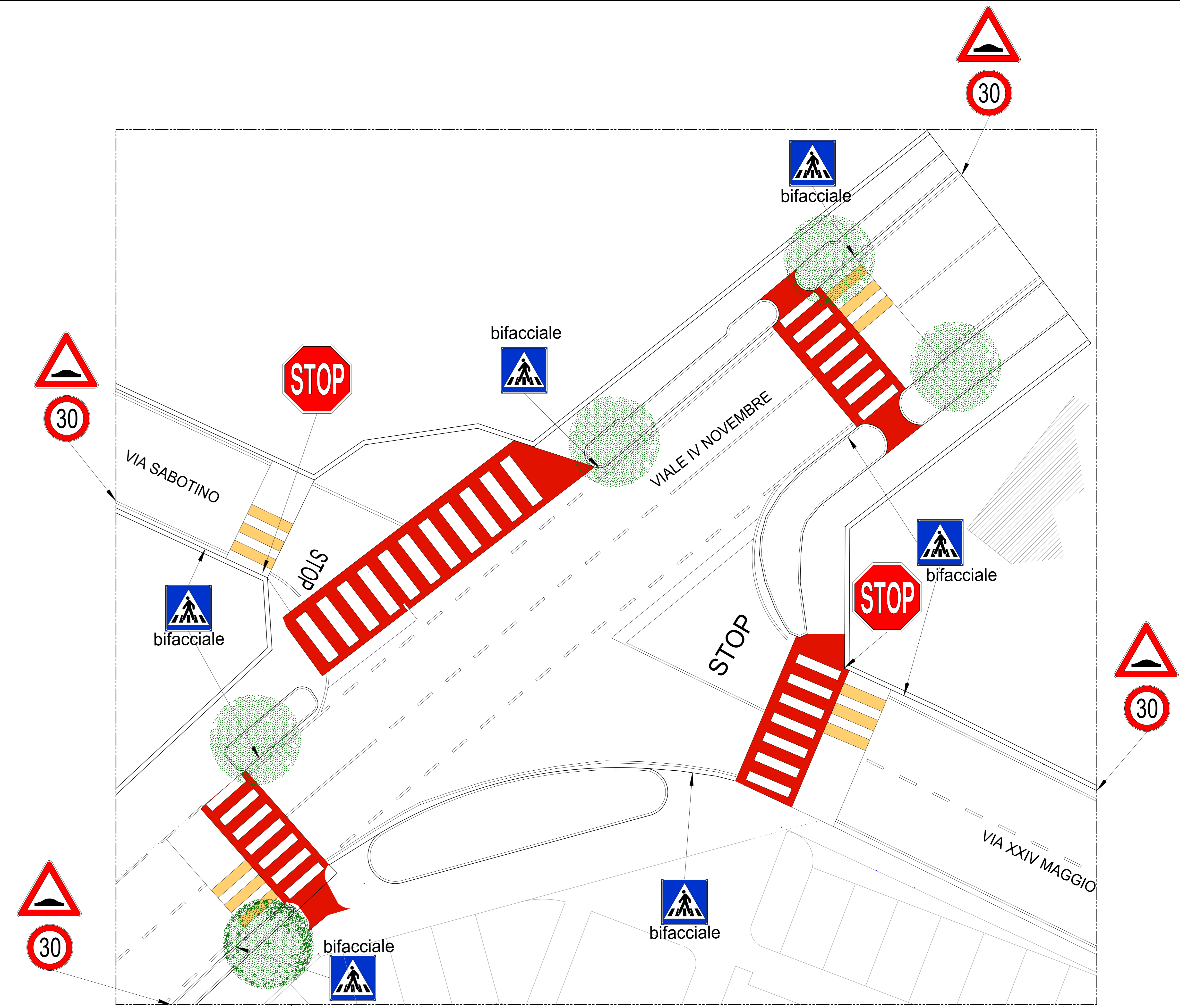
PIANTA DI PROGETTO INTERSEZIONE DA RIQUALIFICARE - SEGNALETICA STRADALE - scala 1:100
